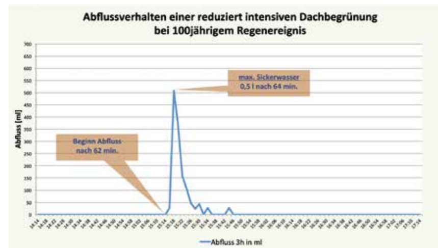
Sickerwasserabfluss einer reduziert intensiven Dachbegrünung bei einem 100-jährigen Regenereignis
