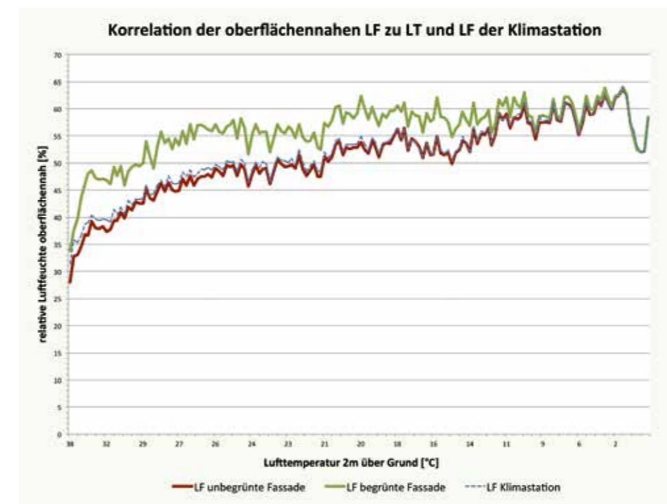
Luftfeuchtigkeit (LF) an einer Grünfassade und an einer Putzfassade in Relation zu den von einer Klimastation aufgetzeichneten Werten der Lufttemperatur und Luftfeuchte
